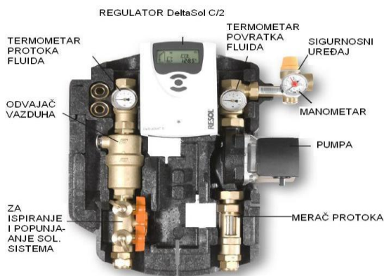
Slika preseka solarne stanice
